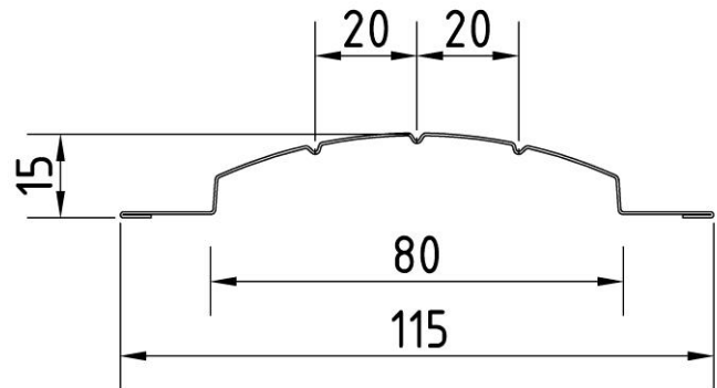
Profil șipcă metalică
